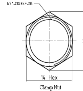
Clamp Nut
