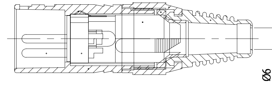
A-A SECTION
